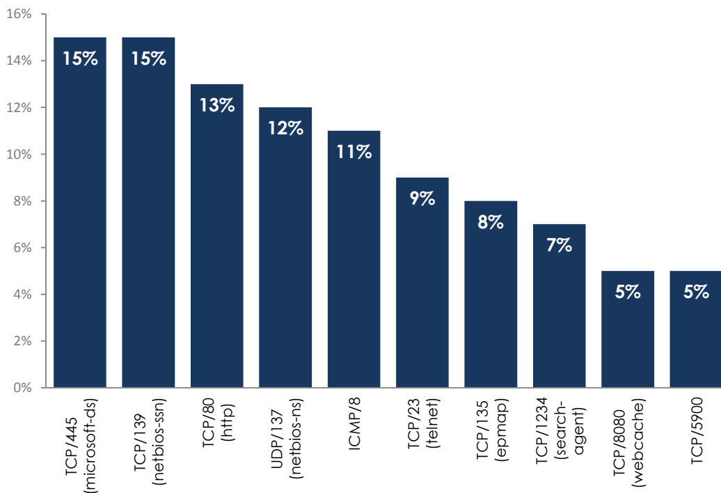
Rysunek 5-13: Najczęściej skanowane porty/usługi w Polsce wg systemu Atlas (odnotowane ilości wystąpień)
