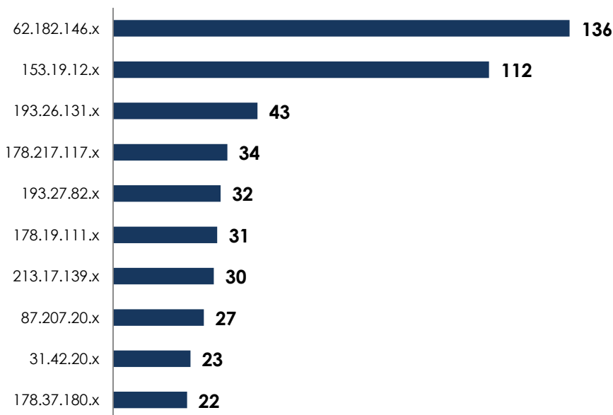
Rysunek 5-14: Najbardziej aktywne hosty w Polsce wg systemu Atlas (ilość wystąpień lub ich sumy dla hostów w jednej podsieci)
