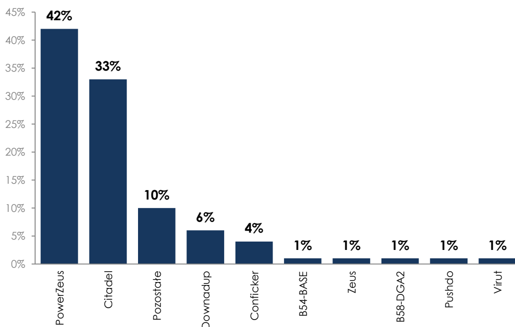
Rysunek 5-7: Udział procentowy ilości przepływów do sieci botnet w roku 2013
